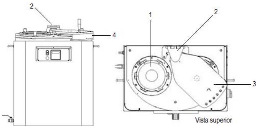
Figura 20: Máquina sorveteira
